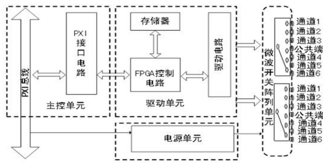
图 6.1 6944F DC ~ 40GHz 1 选 6 微波开关原理框图
