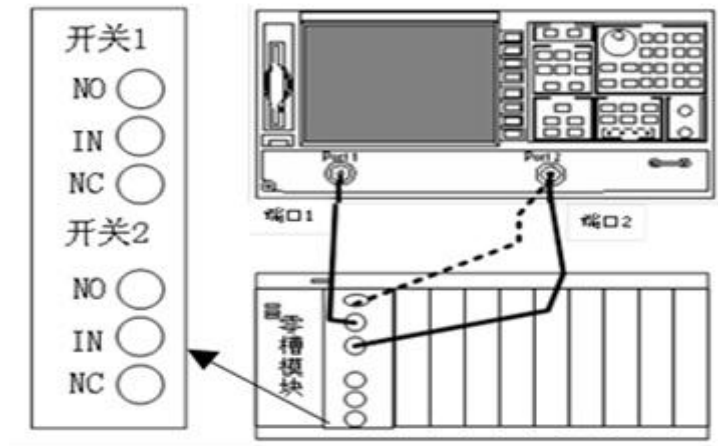
图 7.1 插入损耗测试框图
