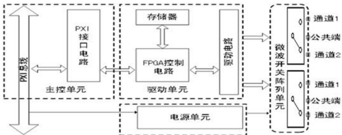
图 6.1 6945F DC ~ 40GHz 1 选 2 微波开关原理框图
