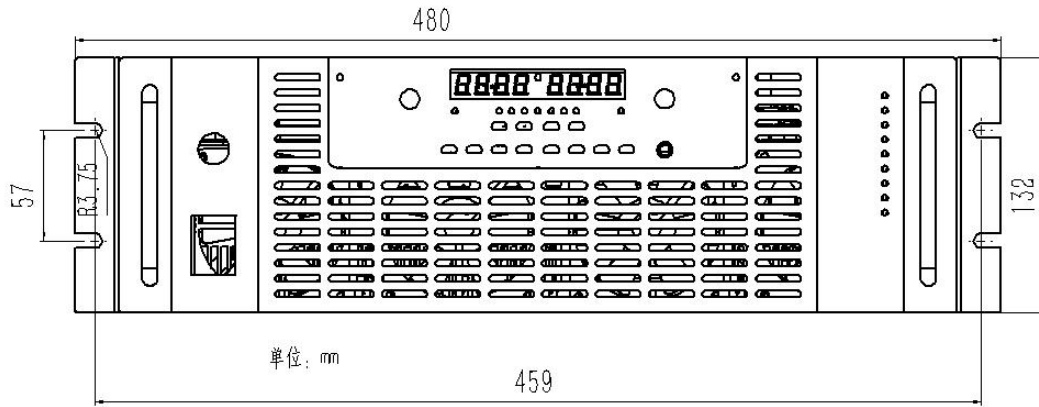
正面尺寸
