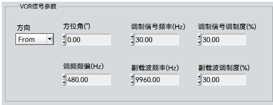
图 3.8 6938AA 信号模拟器方位角设置软件界面
