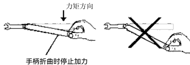
图 3.4 力矩扳手的使用方法
