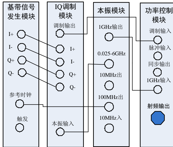
图 3.6 6938AA 信号模拟器前面板
