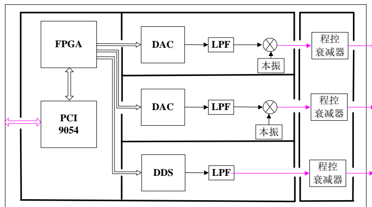
图 6.1 甚高频全向信标模拟器工作原理示意图
