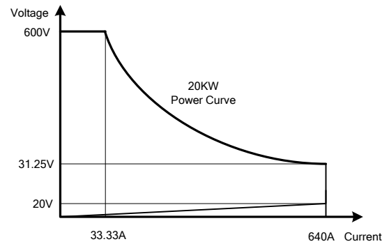
圖 1-1.12 34220A高功率電子負載功率曲線圖
