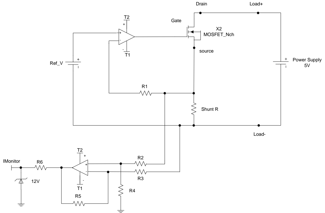
圖 3-5 34000A 系列 I-monitor 等效電路圖
