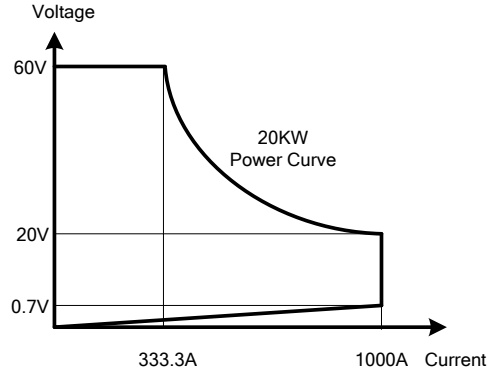
1-1.4 34120A高功率電子負載功率曲線圖
