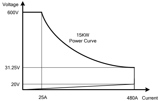
圖 1-1.11 34215A高功率電子負載功率曲線圖
