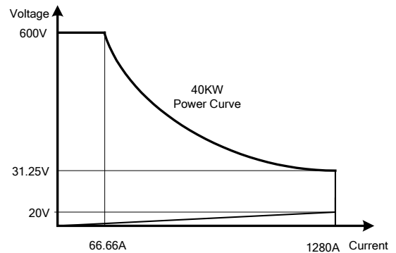
圖 1-1.16 34240A高功率電子負載功率曲線圖
