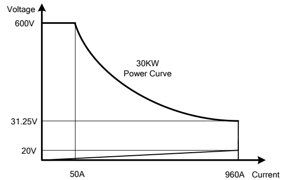
圖 1-1.14 34230A高功率電子負載功率曲線圖
