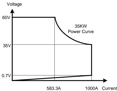
圖 1-1.7 34135A高功率電子負載功率曲線圖
