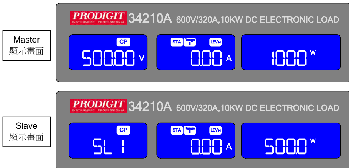
圖 CP Set 1000W
