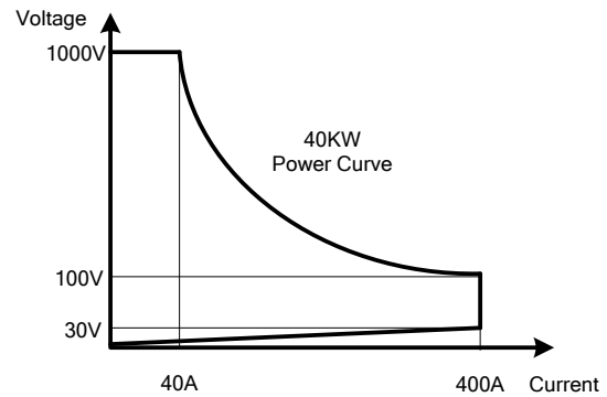
1-1.24 34340A高功率電子負載功率曲線圖
