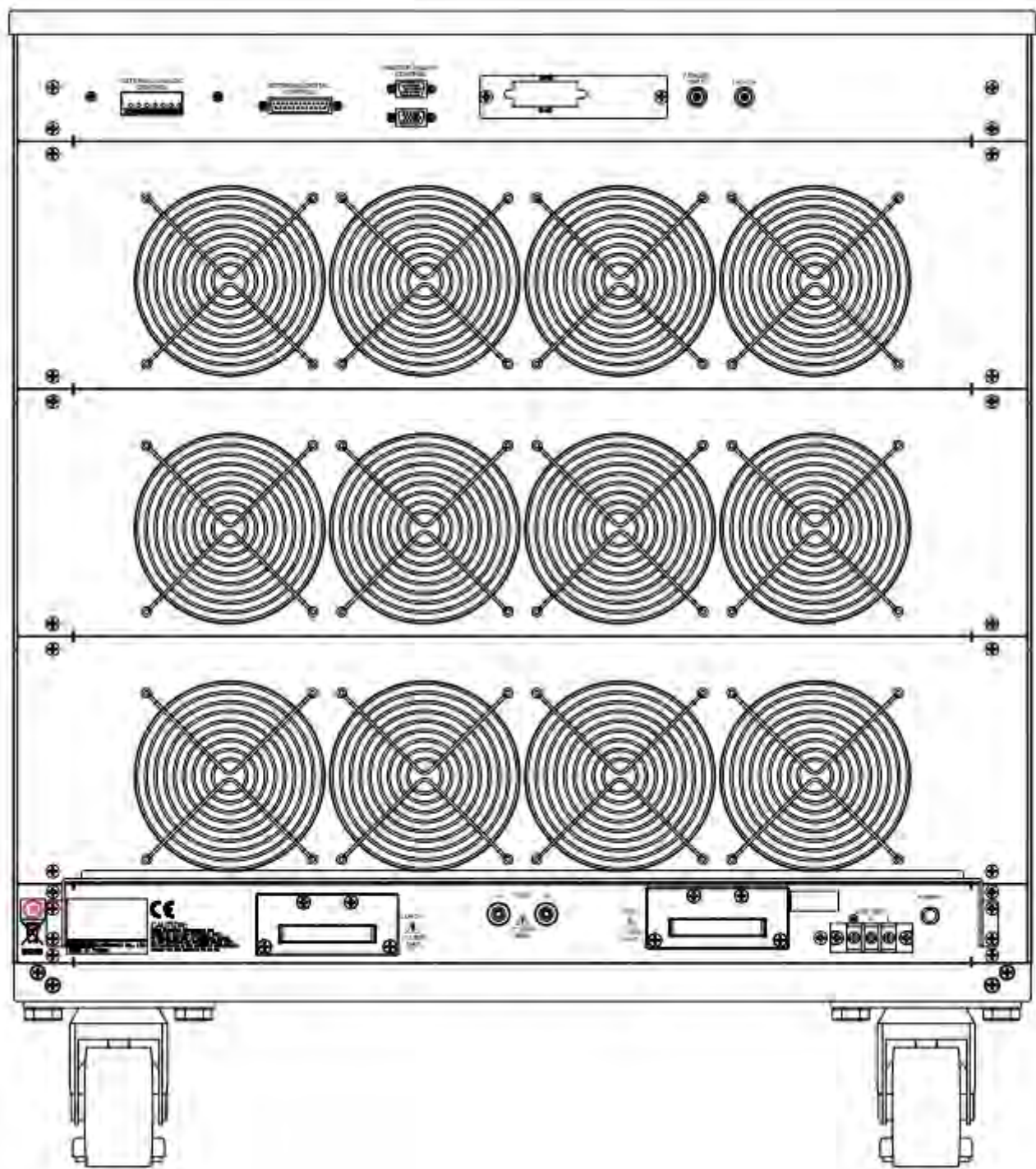
圖 3-2 34000A 系列高功率電子負載後面板圖
