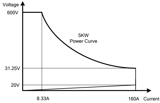
圖 1-1.9 34205A高功率電子負載功率曲線圖
