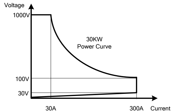
1-1.22 34330A高功率電子負載功率曲線圖
