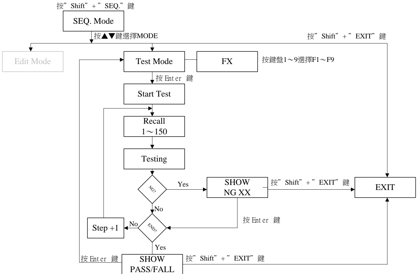
圖 3-10 測試模式操作流程圖
