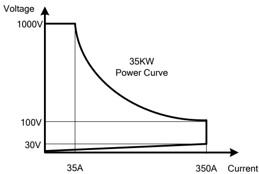
圖 1-1.23 34335A高功率電子負載功率曲線圖
