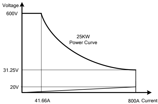
圖 1-1.13 34225A高功率電子負載功率曲線圖
