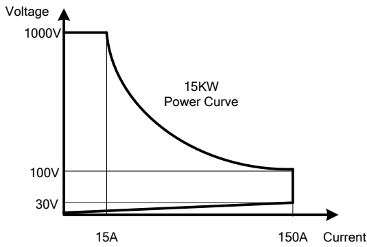
圖 1-1.19 34315A高功率電子負載功率曲線圖
