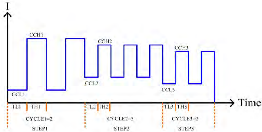
圖 5-17 電池放電測試-TYPE4
