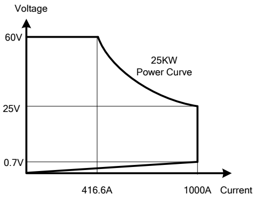
圖 1-1.5 34125A高功率電子負載功率曲線圖
