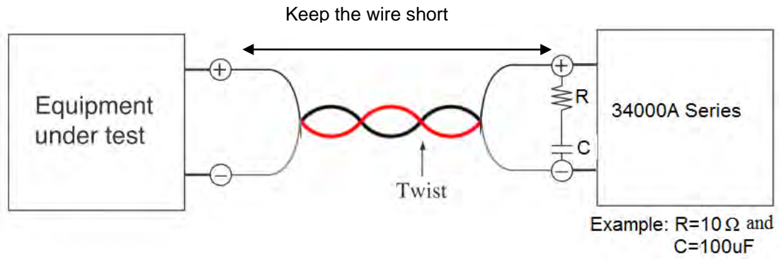
圖 2-10 接線長度
