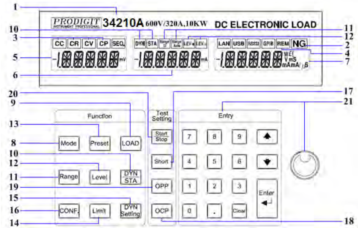
圖 3-3 34000A 系列高功率電子負載之面板圖
