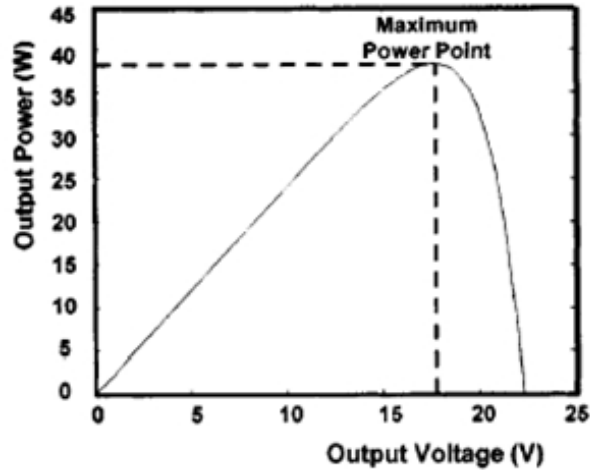
圖 5-11 最大功率點追蹤
