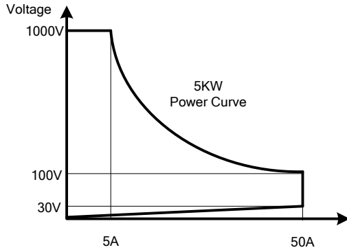
圖 1-1.17 34305A高功率電子負載功率曲線圖
