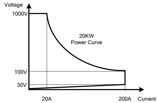
1-1.20 34320A高功率電子負載功率曲線圖
