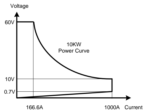
1-1.2 34110A高功率電子負載功率曲線圖
