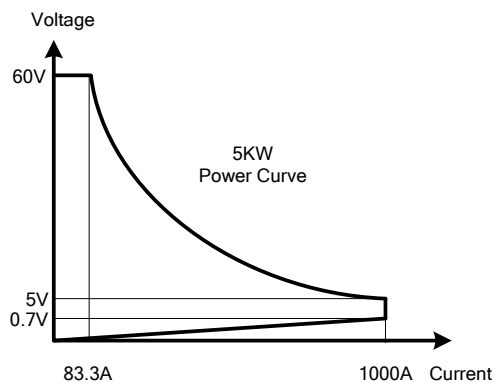
圖 1-1.1 34105A高功率電子負載功率曲線圖
