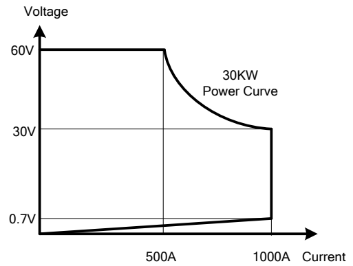
1-1.6 34130A高功率電子負載功率曲線圖
