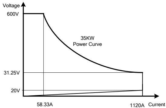
圖 1-1.15 34235A高功率電子負載功率曲線圖
