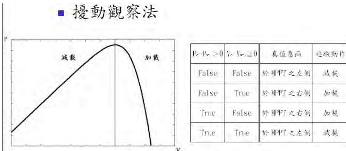
圖 5-12 擾動觀察法動作方式
