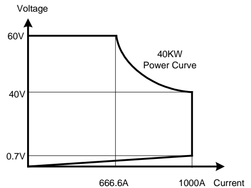
1-1.8 34140A高功率電子負載功率曲線圖
