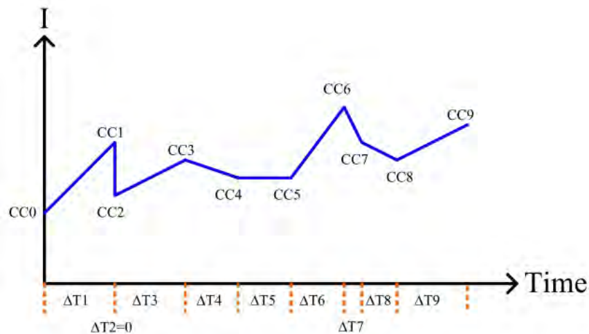
圖 5-18 電池放電測試-TYPE5
