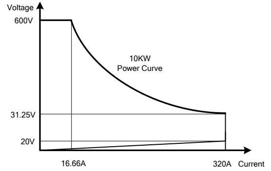
圖 1-1.10 34210A高功率電子負載功率曲線圖
