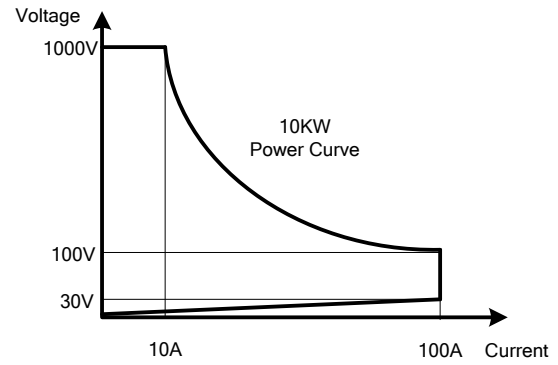
1-1.18 34310A高功率電子負載功率曲線圖
