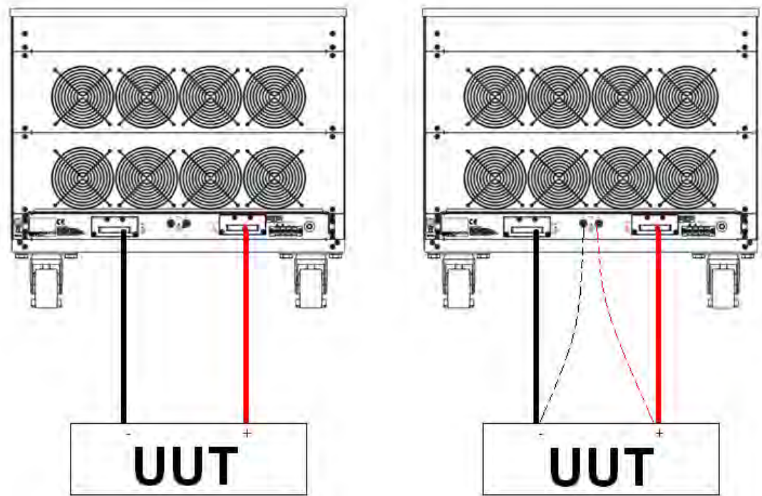
圖 3-4 典型 34000A 系列高功率電子負載連接方式
