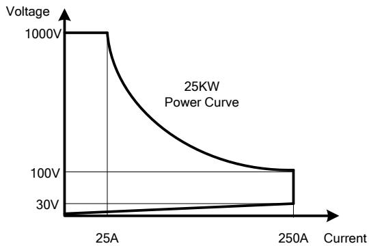
圖 1-1.21 34325A高功率電子負載功率曲線圖
