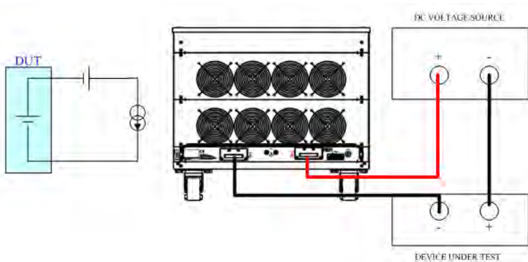
圖 5-11 高功率電子負載最低工作電壓為 0V 時的連接圖
