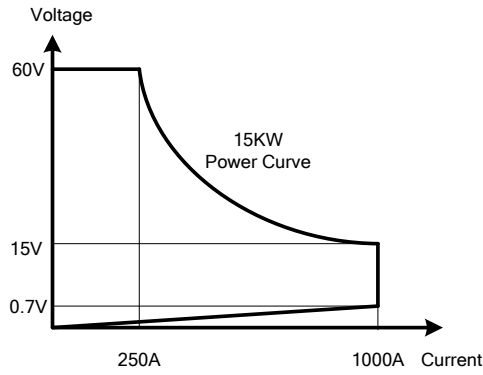
圖 1-1.3 34115A高功率電子負載功率曲線圖
