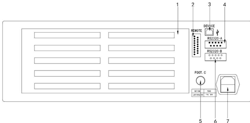
图 2-2 对 UC6601 后面板进行了简要说明
