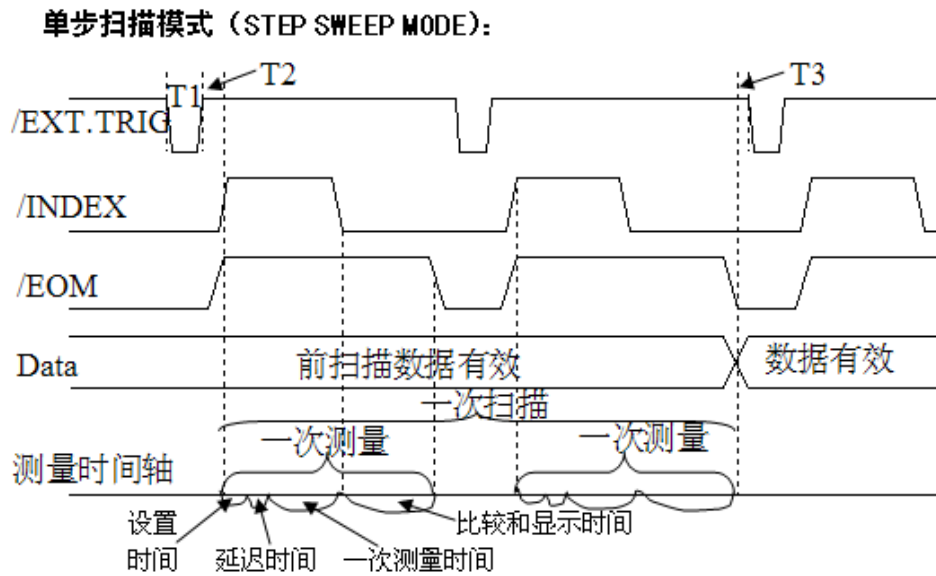
图 7-4 列表扫描时序图解
