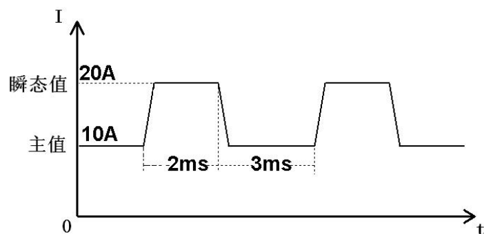
图 5-28 连续方式
