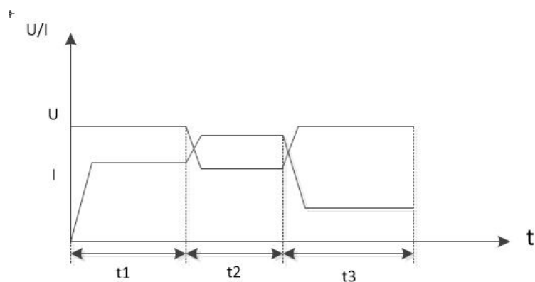
图 5-38 自动测试
