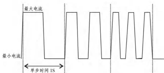
图 5-20 动态扫描
