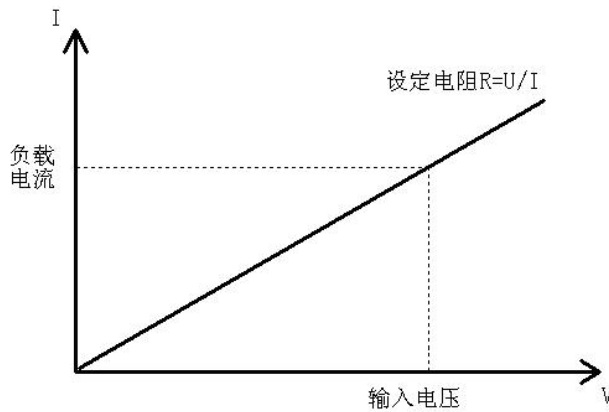
图 5-9 恒电阻模式
