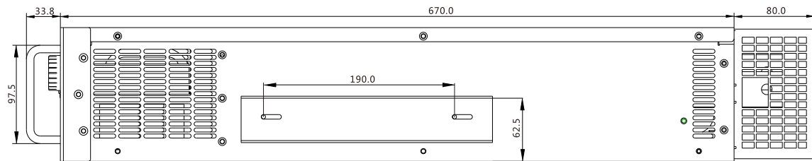
图 3-2 从机机箱侧视尺寸 (mm)
