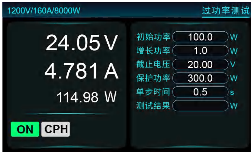
图 5-46 运行过功率测试
