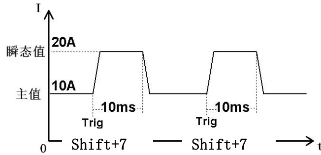
图 5-27 脉冲方式
