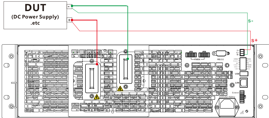
图 3-15 采样连接
