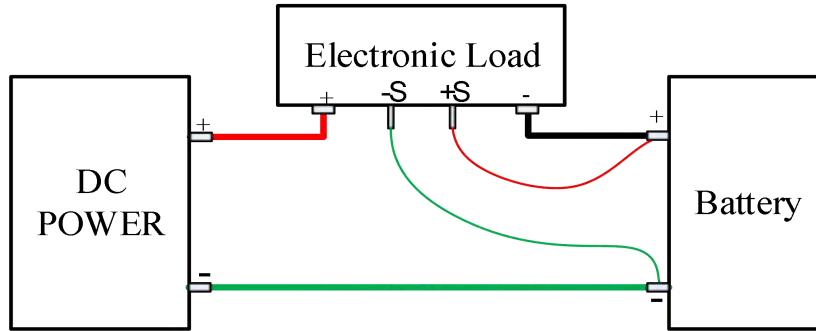
图 5-40 充电测试接线示意图
