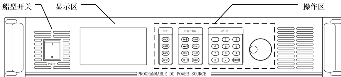
图 5：前面板
