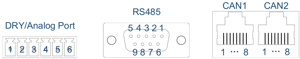
图 2: 接口
