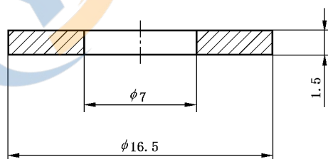
e) PTFE 部件 II 切面侧视图
