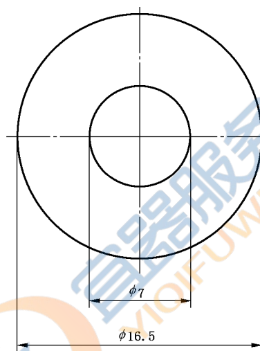
d) PTFE 部件 II 俯视图
