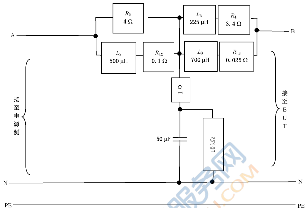
图 B.3 适用于 16 A 电流及以下测量的人工电源网络
