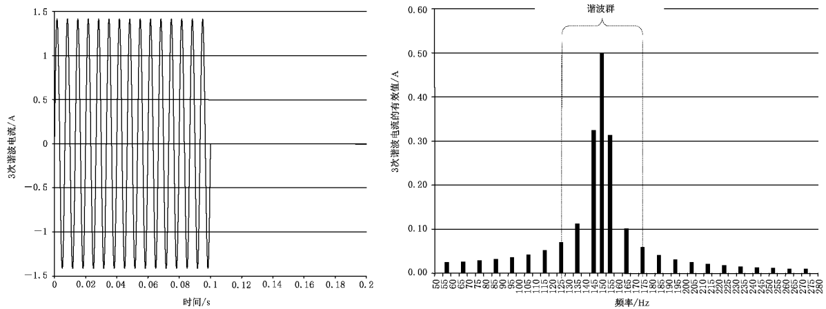
图 C.3 某微波器具波动的 3 次谐波电流
