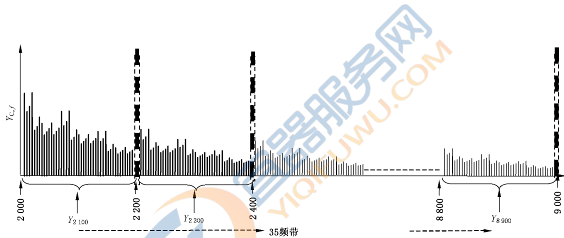
图 B.1 50 Hz 电力系统中 40 次谐波频率以上至 9 kHz 的频带范围内测量示意图
