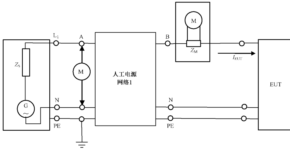
a) 单相测量布置
