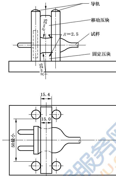
图 38 25.4 的检验耐热性能的压缩试验装置
