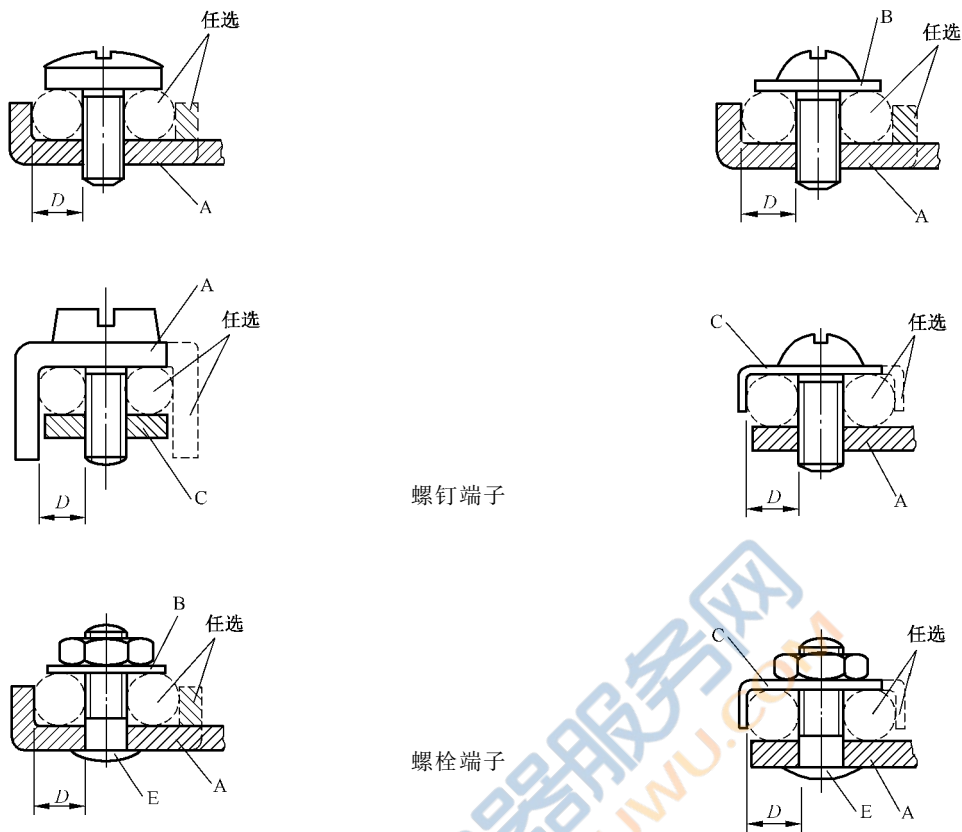
a) 不要求垫圈或夹紧板的螺钉/螺栓
