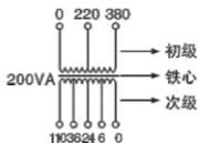
图4 连续式中间带抽头绕组
