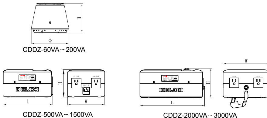
CDDZ系列交流电源变压器外形及安装尺寸
