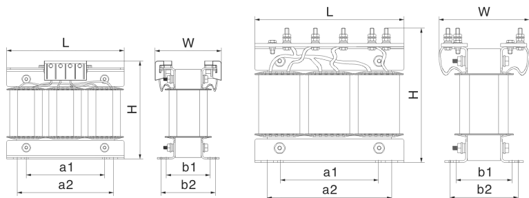
SBK-10kVA及以下
