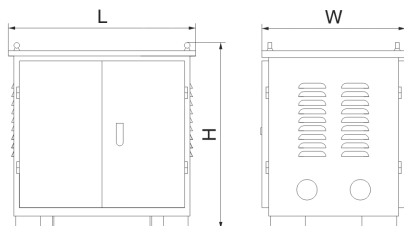
SBK-80kVA及以上
