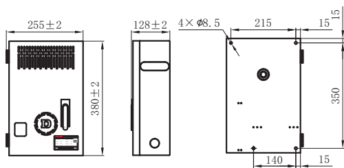
CDQB-1000W~2000W墙暖电源控制箱
