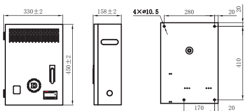
CDQB-2500W~5000W墙暖电源控制箱
