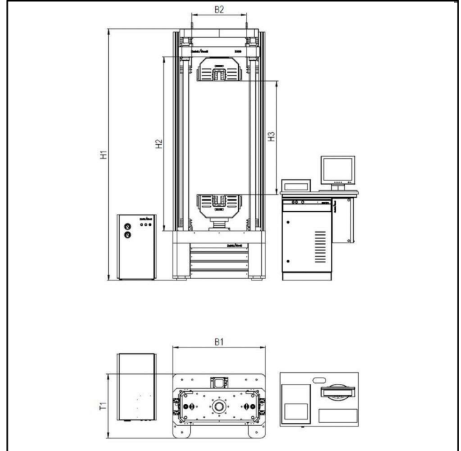
Zeichnung: Z400E mit Hydraulik-Probenhalter
