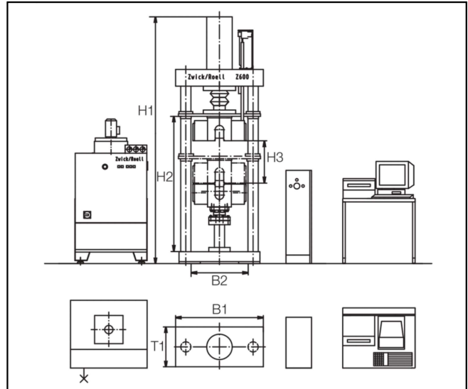
Zeichnung der ZwickRoell Z600H mit Hydraulik-Probenhalter
