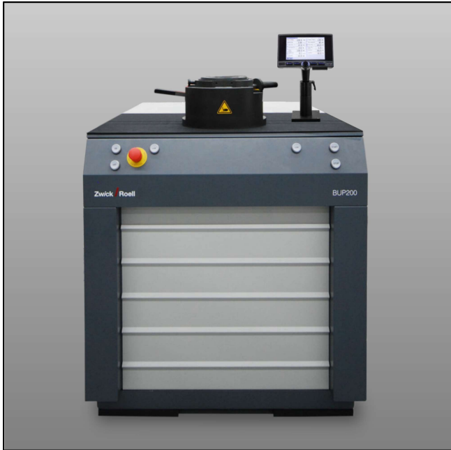
Blechumform-Prüfmaschine BUP 200
