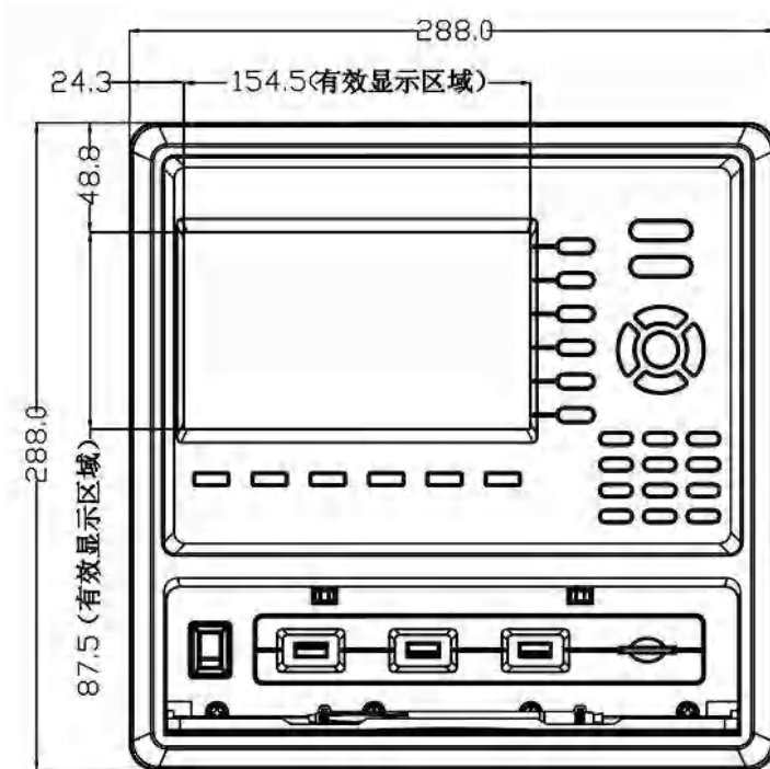
外形尺寸：288×288×200mm (长×宽×深)
