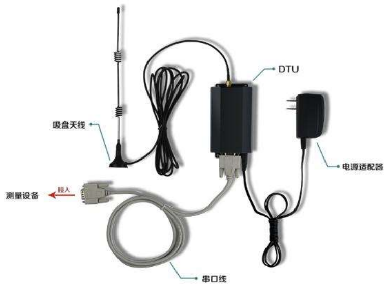
图 7-14 DTU-无线短信报警器
