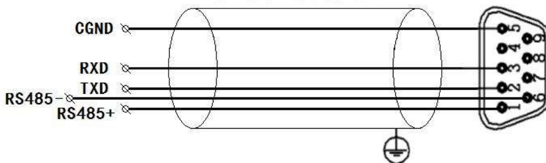
串口通讯接线说明
