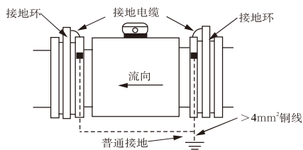
B、塑料管道接地
