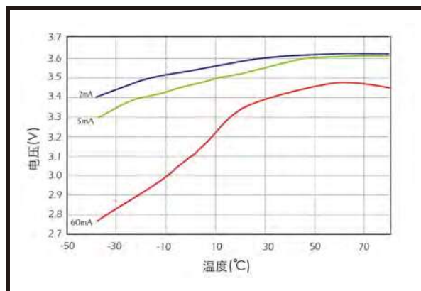
2、在不同放电电流和温度条件下的平稳电压曲线图（在放电的稳定阶段）
