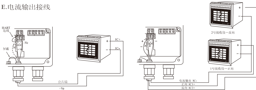
标准型电流输出接线图
