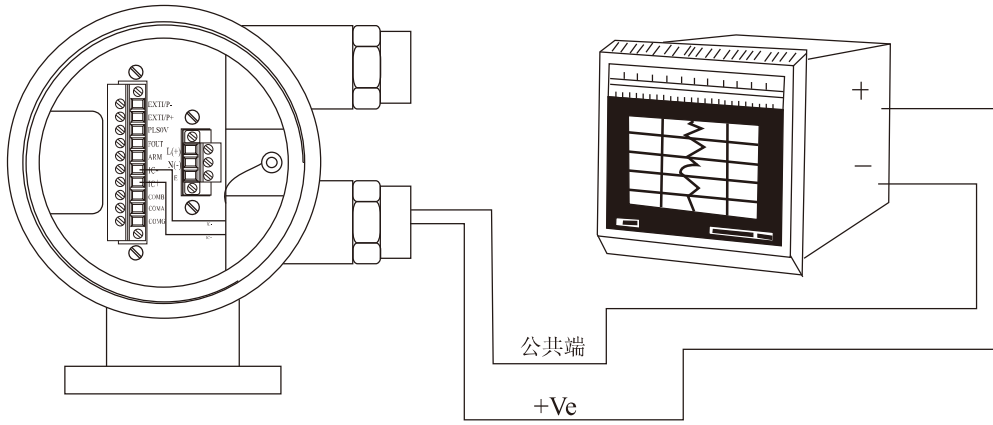
标准型电流输出接线图
