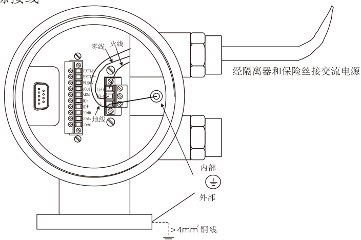
交流供电电源连接图 (AC220V)
