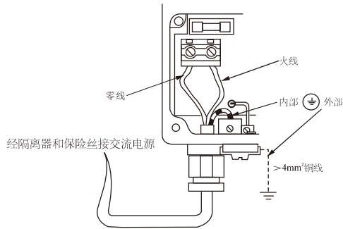
交流供电电源连接图 (AC220V)
