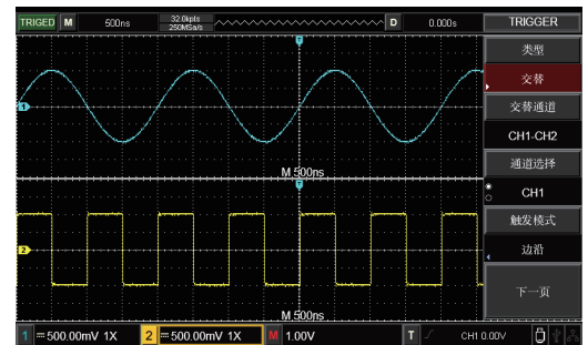
4 多种触发功能(图为交替触发), 适用于复杂测试环境
