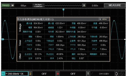
3 多种波形参数自动测量
