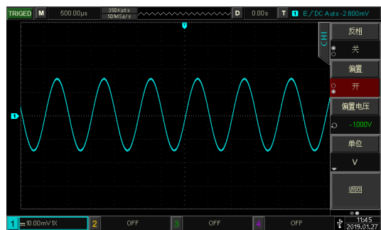
图 2-4 -1V 偏置
