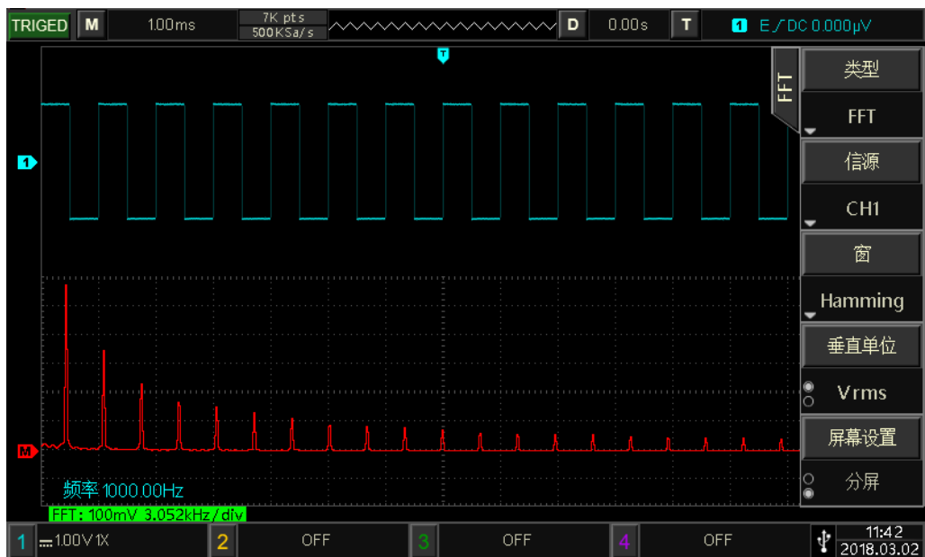
图 5-1 FFT 频谱
