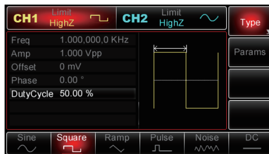
2 占空比为50%的方波信号
