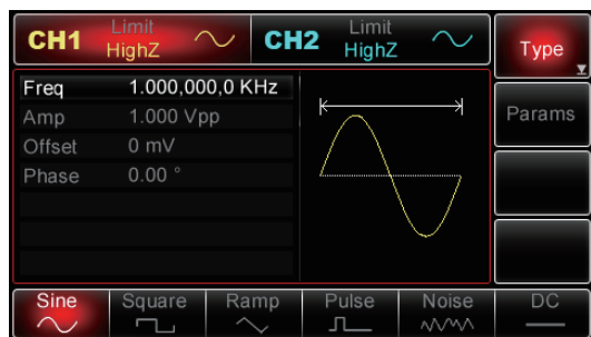
1 双通道有多种基本波形可选择
