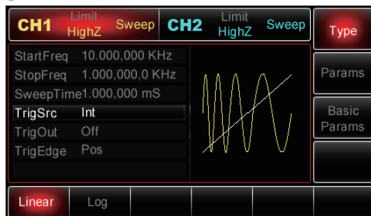
5 线性和对数扫描信号
