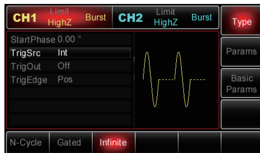
6 三种猝发模式
