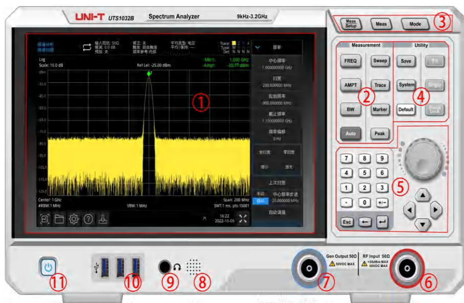
图 1-1: 前面板
