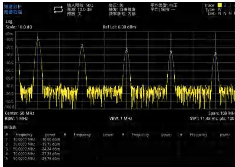
图 4-3: 峰值表
