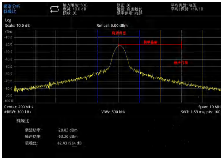
图 5-7：载噪比测量
