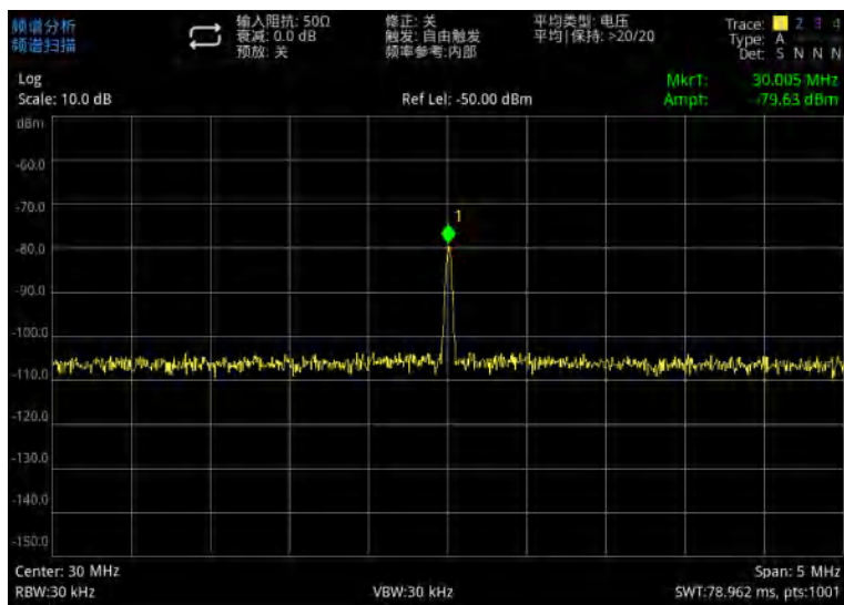
图 3-14: 迹线平均
