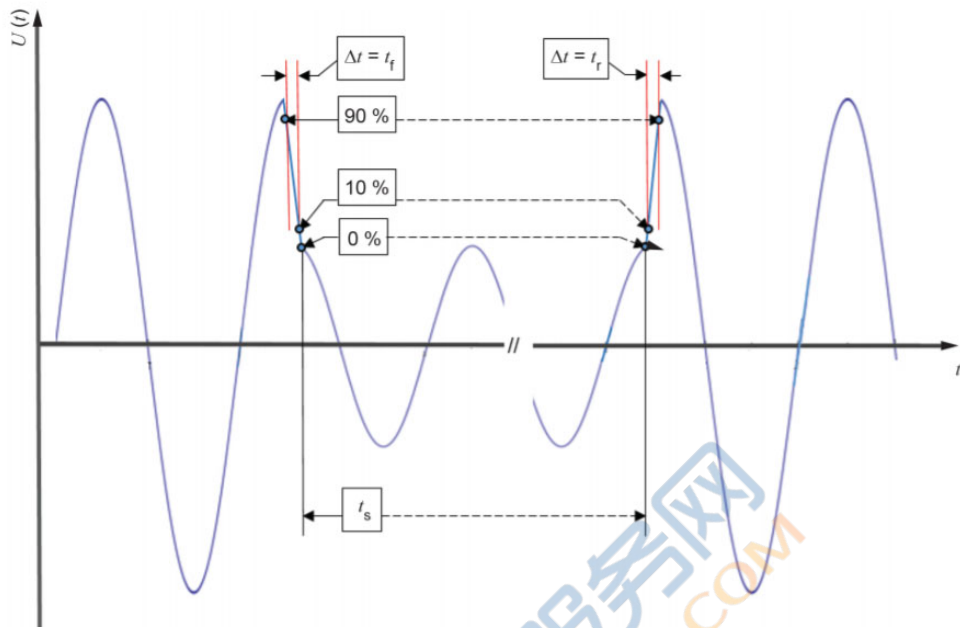
图1 电压暂降示例
