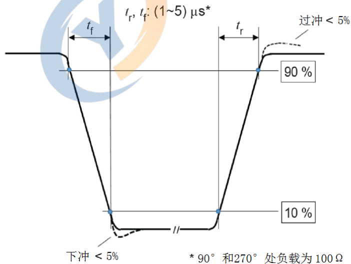
图3 电压上升和下降时间细节图
