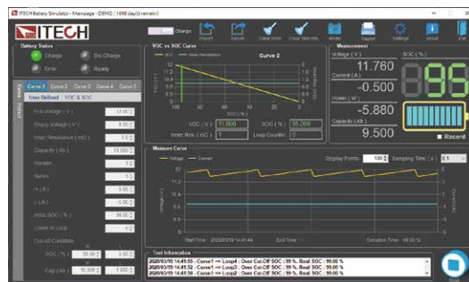
BSS2000电池模拟软件测试界面
