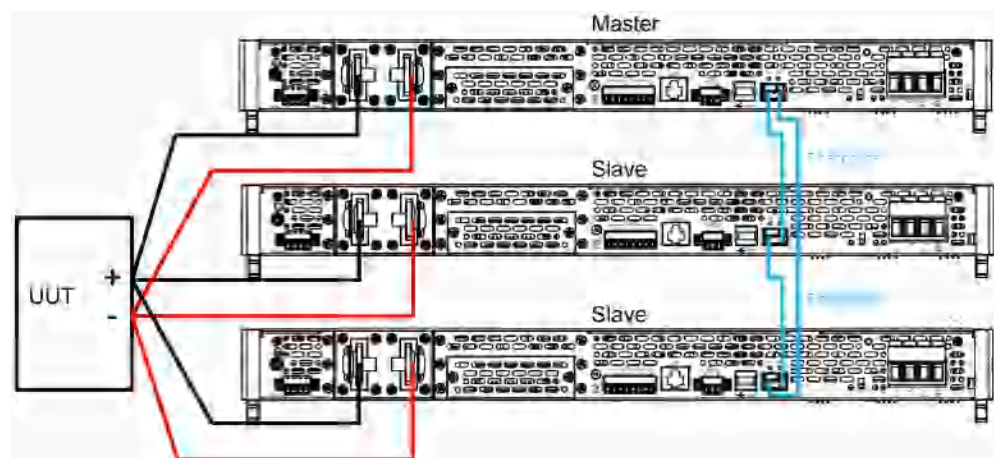
图 5-1 线路连接图
