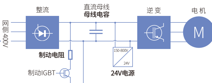
集成式变桨系统拓补图
