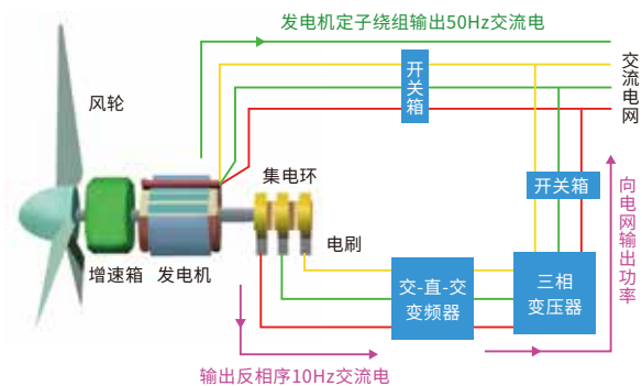
双馈式风力发电机系统原理图
