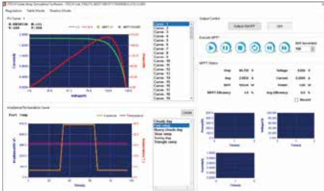
模拟不同温度/照度下的I-V曲线
