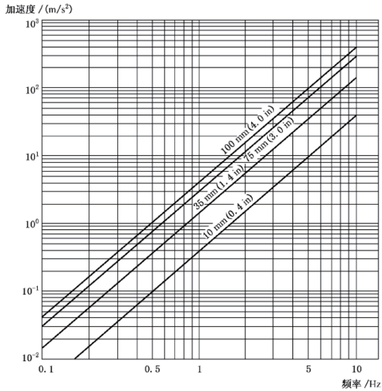
图 2 采用高交越频率(58 Hz~62 Hz)时的振动幅值与频率的关系图
