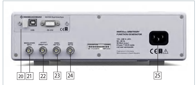
Abb. 2.2: Geräterückseite R&S®HMF2550
