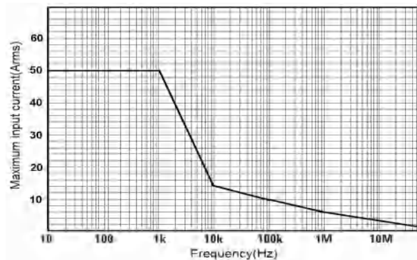
图 5 HCP8050 最大测量电流 VS 频率曲线
