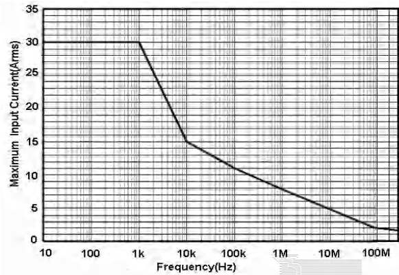
图 2.d HCP8030H 最大测量电流 VS 频率曲线
