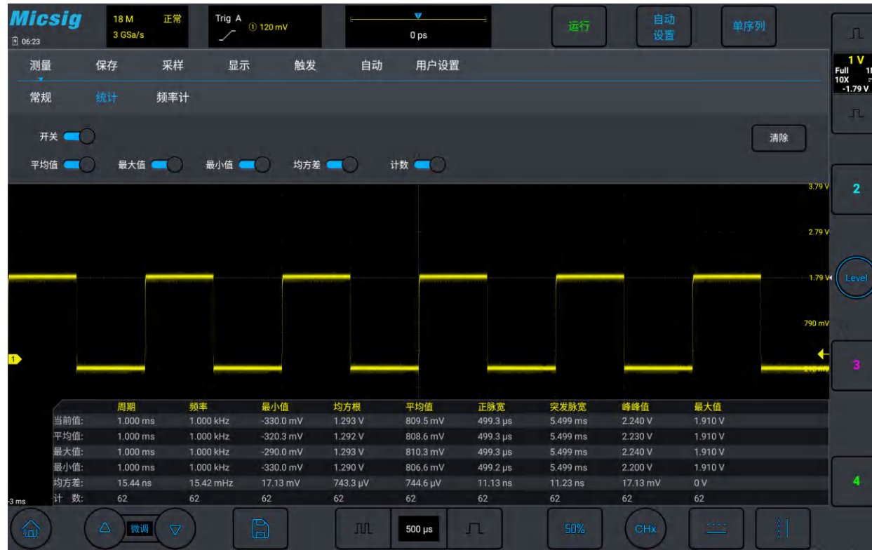
图6-8 统计菜单
