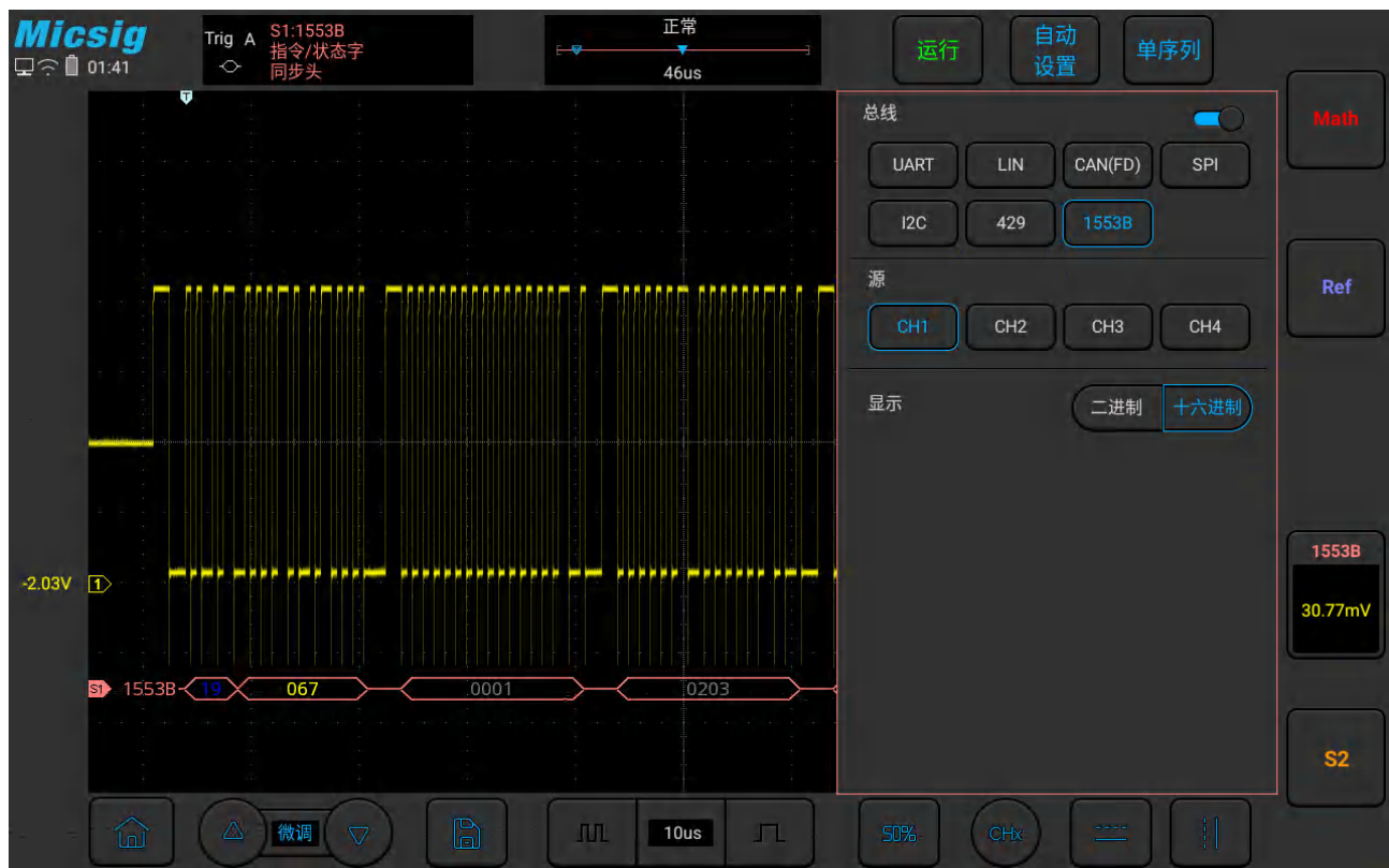
图11-30 1553B 总线配置菜单
