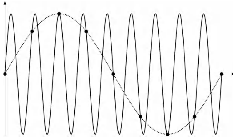
图10-1 混叠
