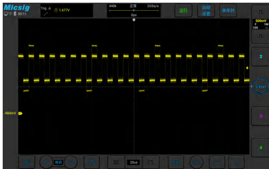
图5-3 周期信号中有异常信号
