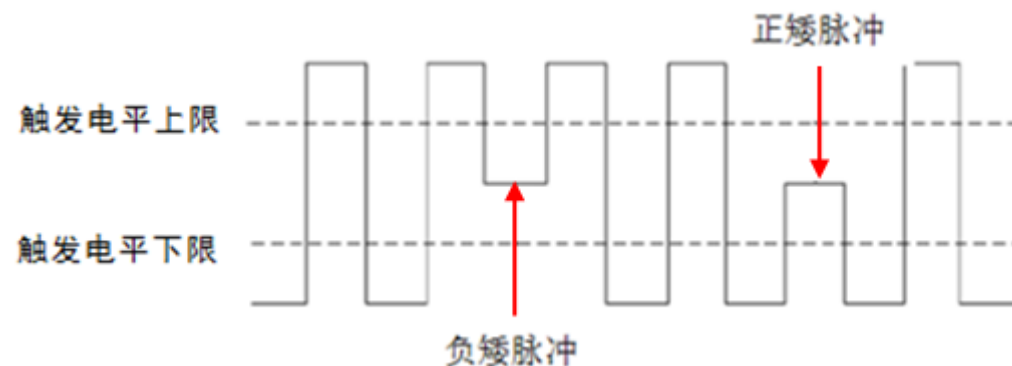
图5-24 欠幅触发
