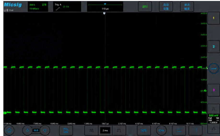
图10-6 带毛刺的波形，正常采样模式
