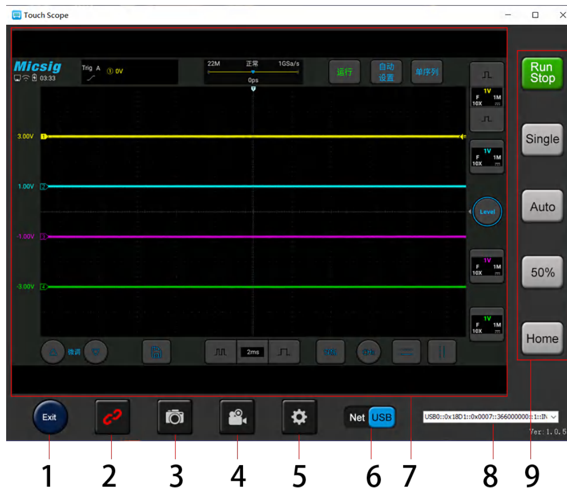
图13-2 上位机界面
