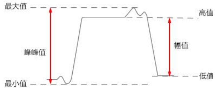
图6-7 电压测量
