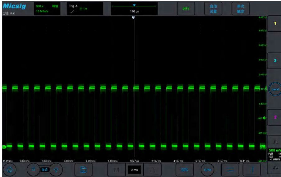
图10-5 带毛刺的波形，峰值采样模式
