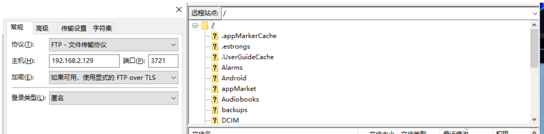
图12-15 FileZilla
