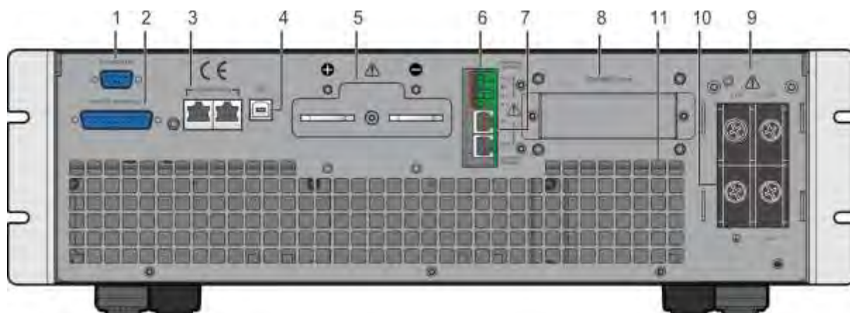
圖 1-7 62000H 系列具太陽能電池陣列模擬機型的後背板
