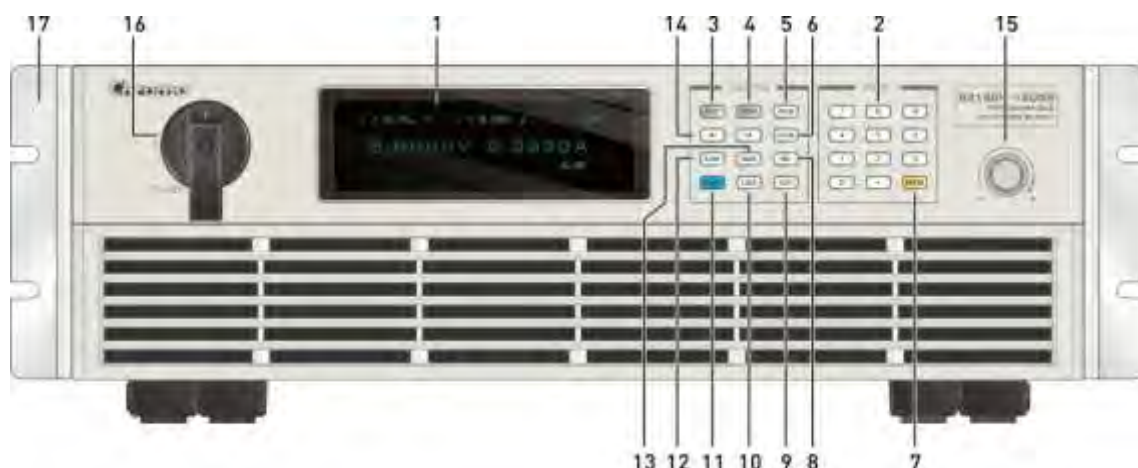
圖 1-6 62180H-1800S 具太陽能電池陣列模擬機型的前面板
