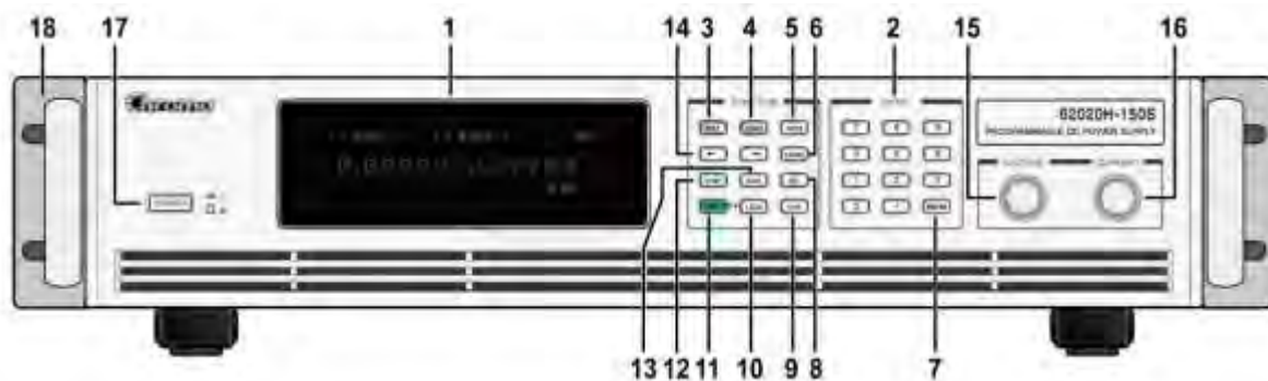
圖 1-5 62020H-150S 具太陽能電池陣列模擬機型的前面板
