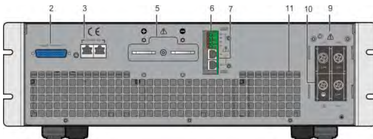
圖 1-8 A620027/A620028 SLAVE 機型後背板
