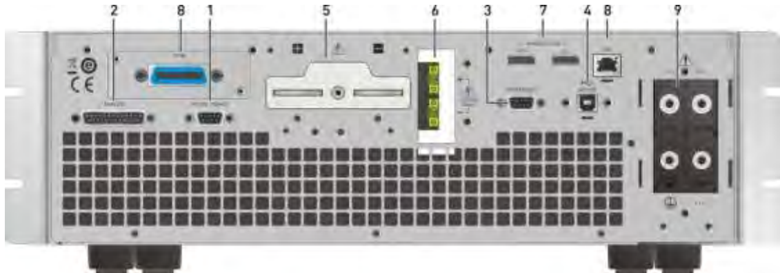
圖 1-10 62180H-1800S 具太陽能電池陣列模擬機型的後背板
