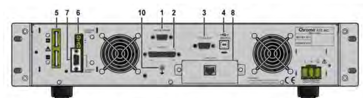
圖 1-9 62020H-150S 具太陽能電池陣列模擬機型的後背板
