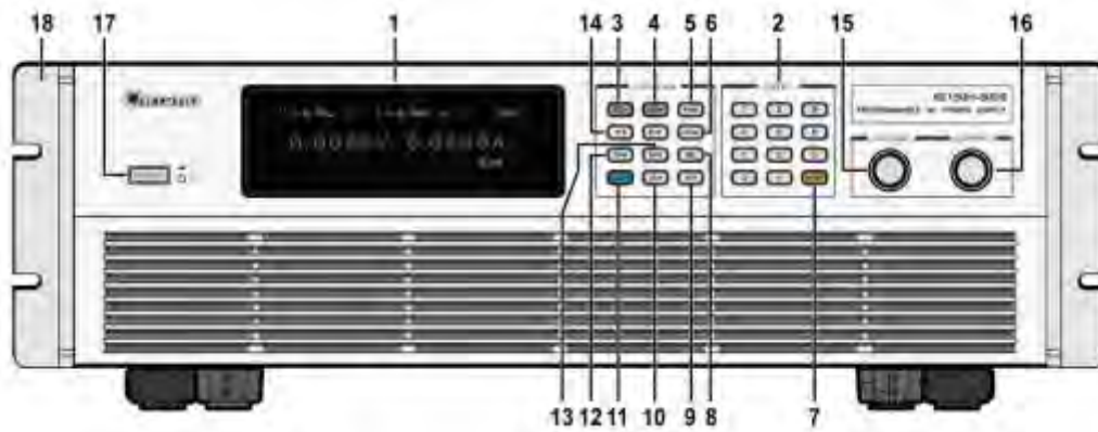
圖 1-3 62000H 系列具太陽能電池陣列模擬機型的前面板
