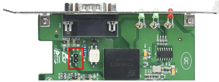
图 2.2 终端电阻选择示意图
