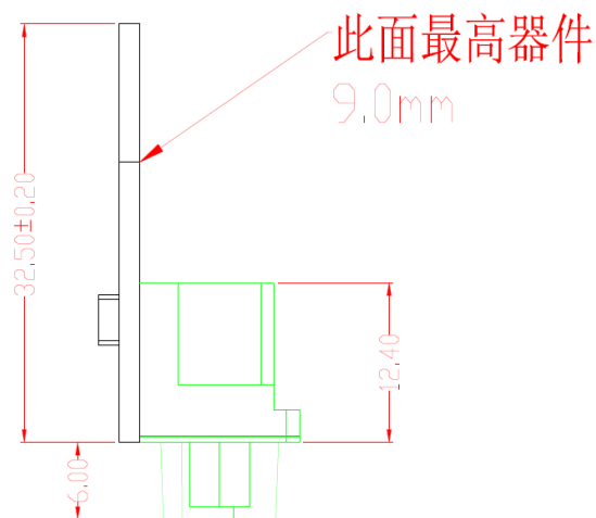
图 7.2 PACK 板尺寸
