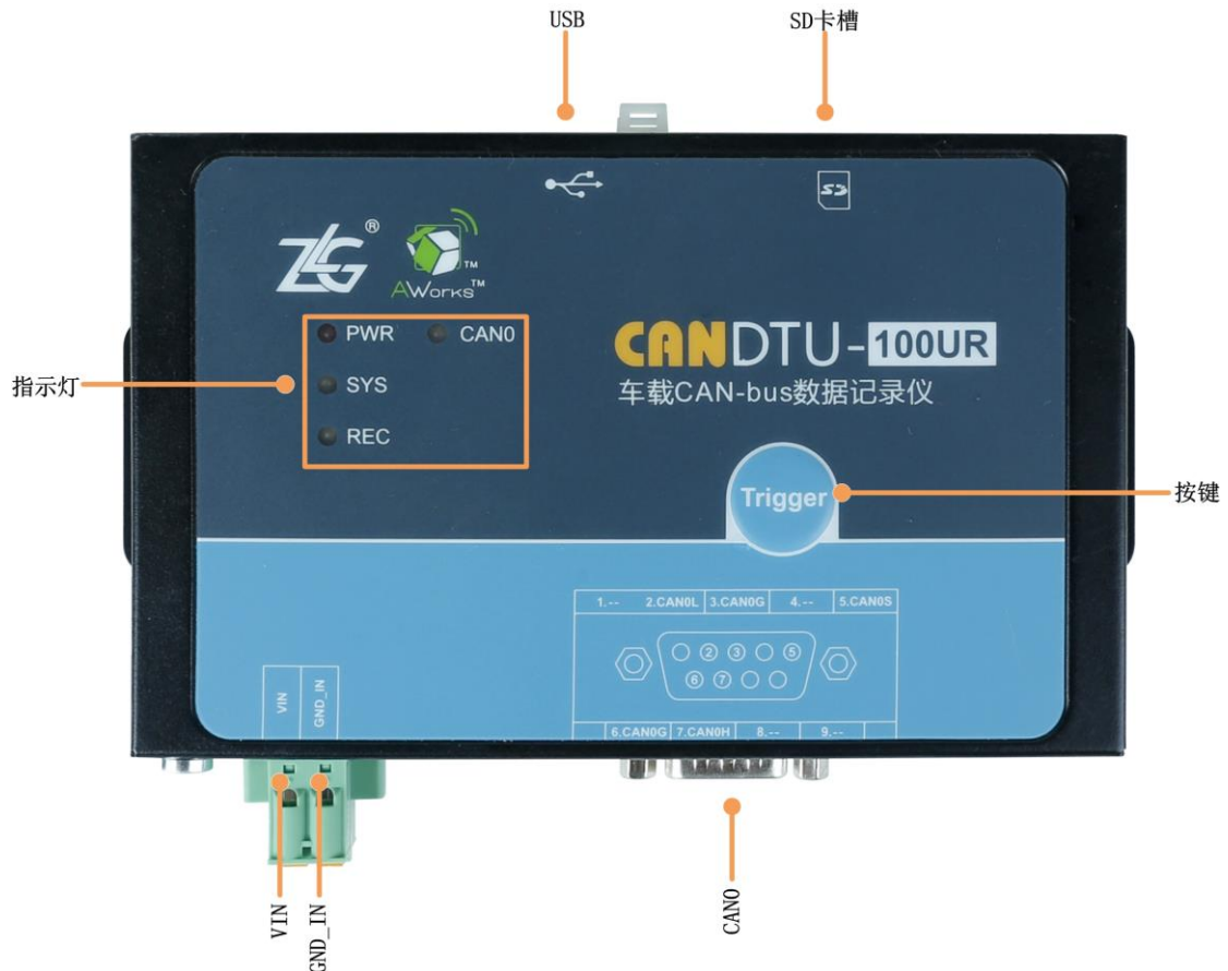
图 3.1 面板布局
