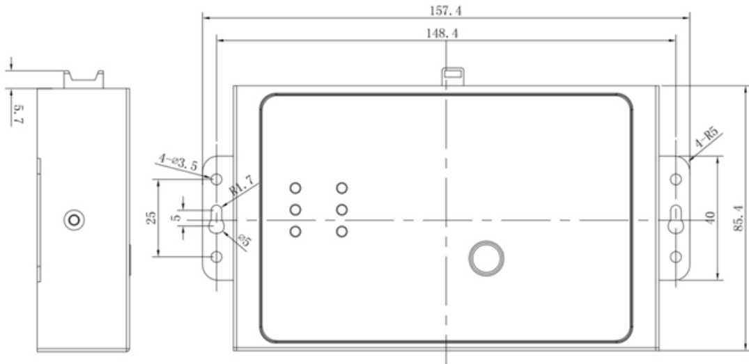
图 2.1 机械尺寸
