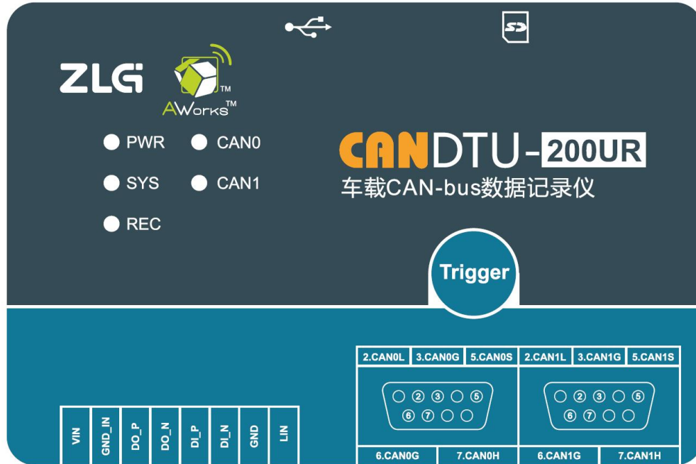
图 3.1 面板布局
