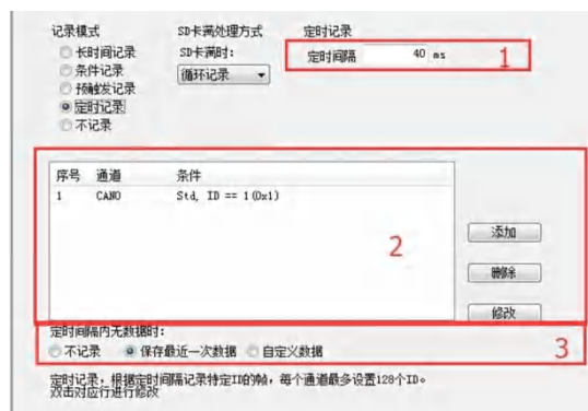
图 4.16 定时记录
