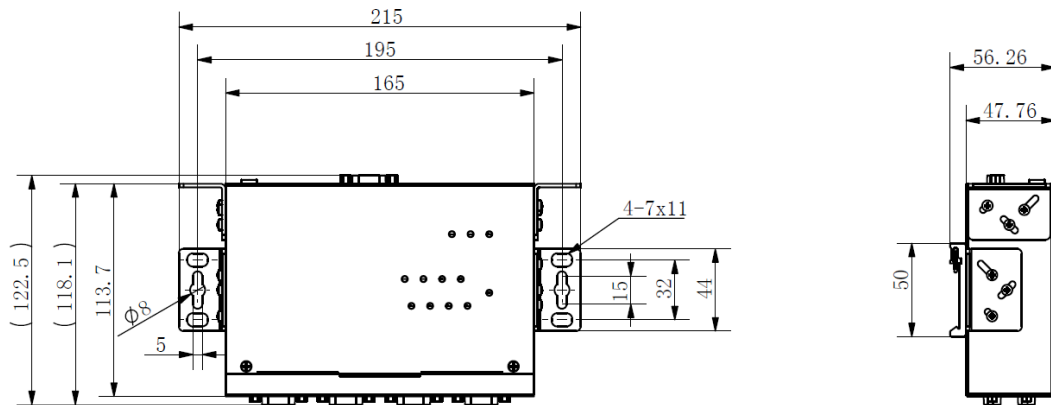
图 1.1 CANhub-AS5 安装机械尺寸图
