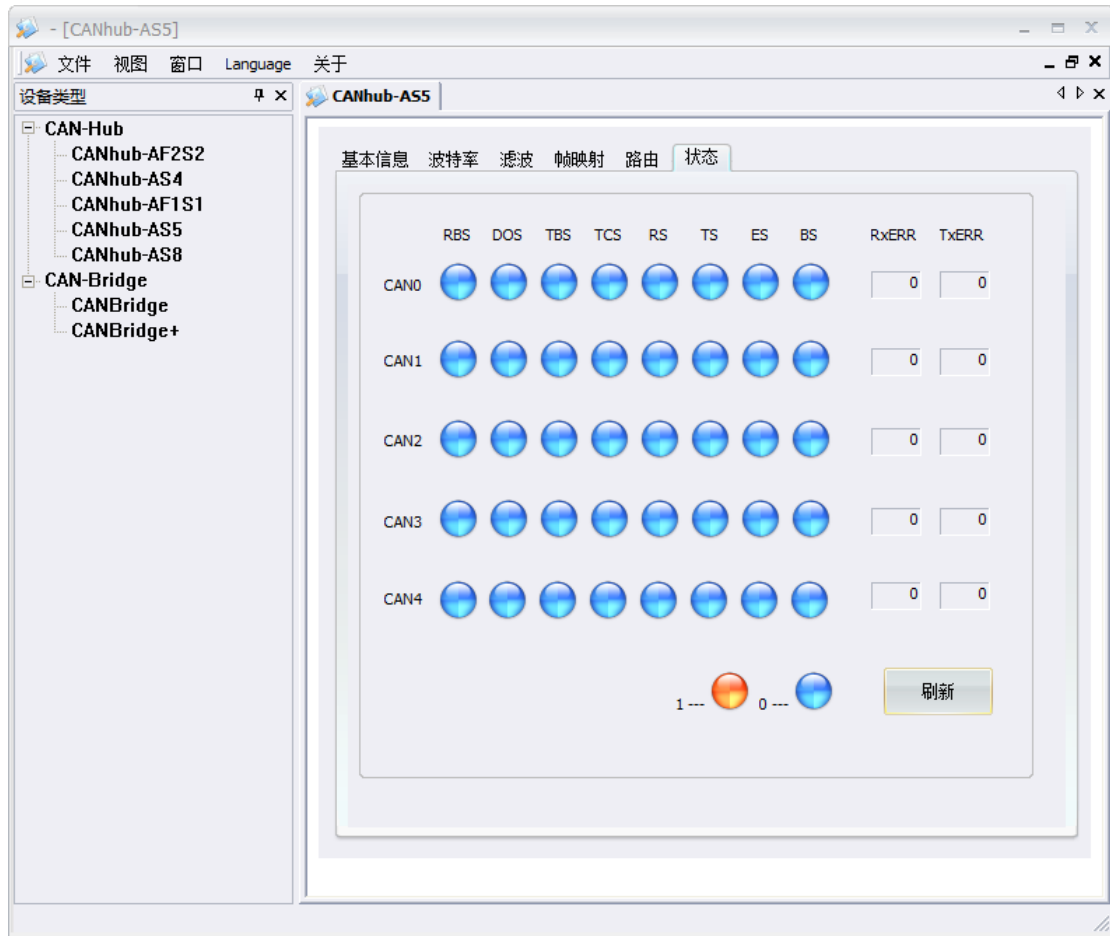
图 4.15 各通道状态
