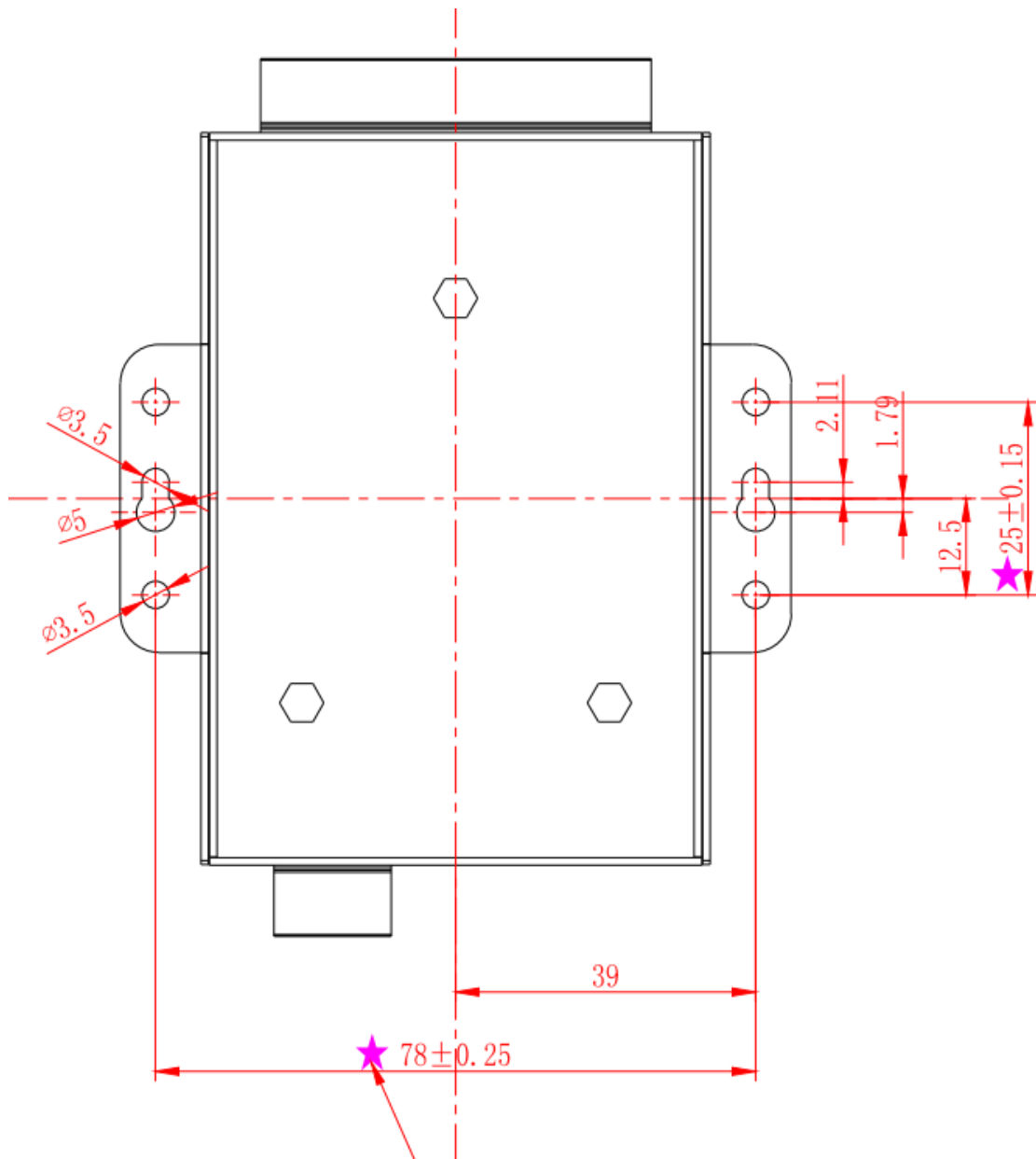
图 7.1 产品尺寸图
