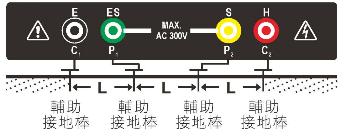
土壤電阻率量測
