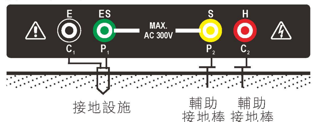
接地電阻量測
