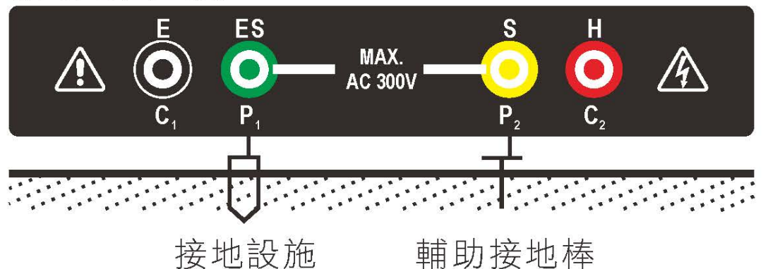
接地電壓量測
