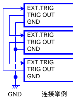
连接举例
