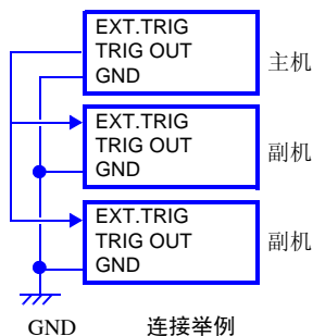
连接举例
