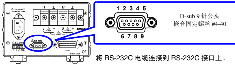
RS-232C 接口
