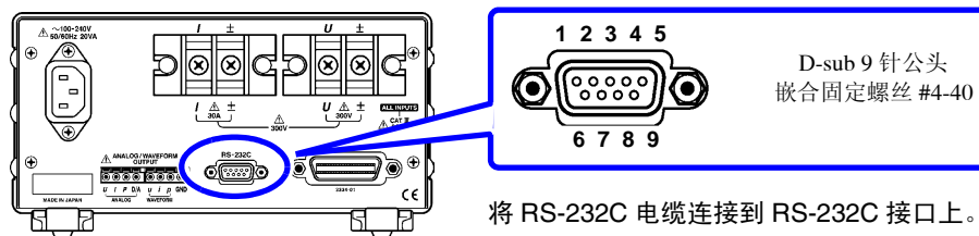
RS-232C 接口
