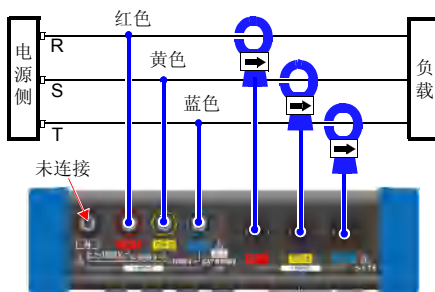
三相 3 线 (3P3W3M) 3 功率表法
