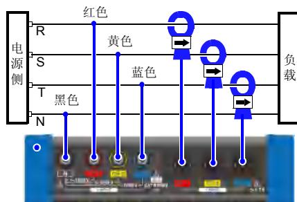
三相 4 线 (3P4W)
