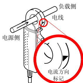
9660 钳式传感器
