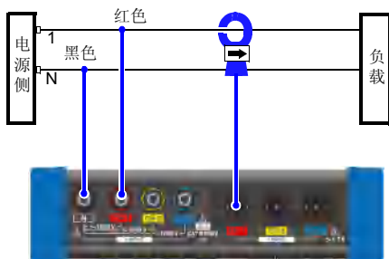
单相 2 线 (1P2W)
