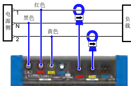
单相 3 线 (1P3W)
