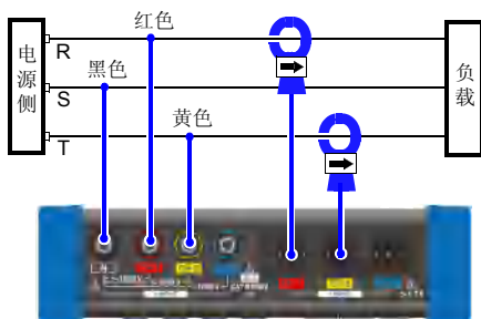
三相 3 线 (3P3W2M) 2 功率表法
