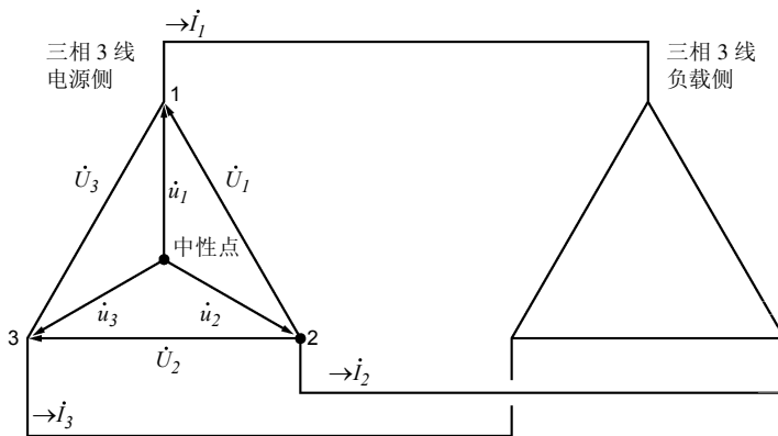
三相 3 线线路的类似回路
