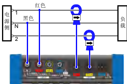
三相 3 线 (1P3W1U) (1 电压测量)
