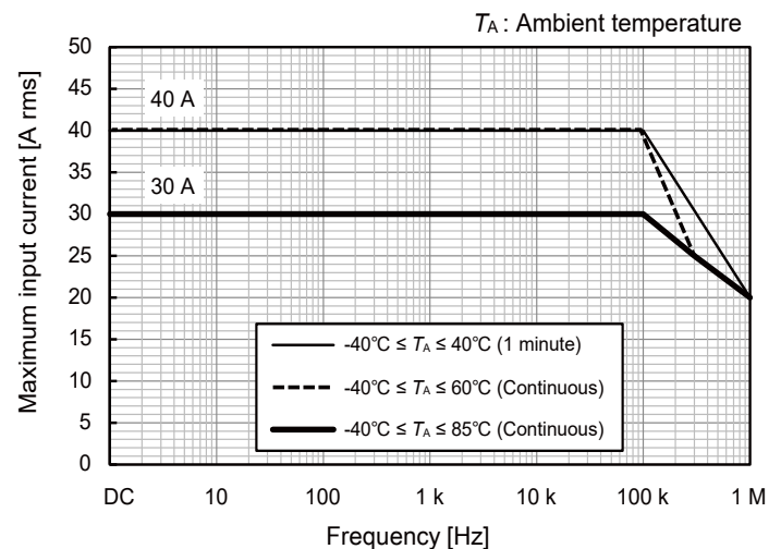
图 1. 频率额定值降低特性*
