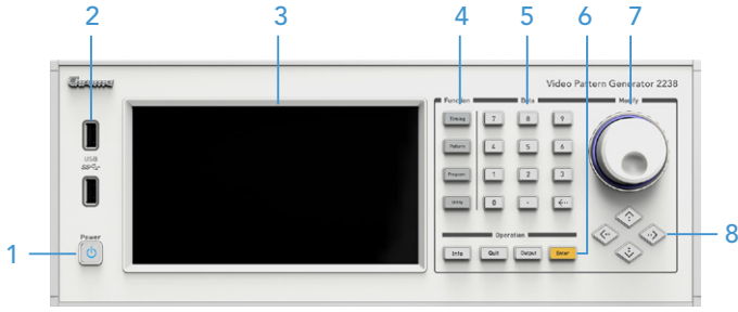
前面板
