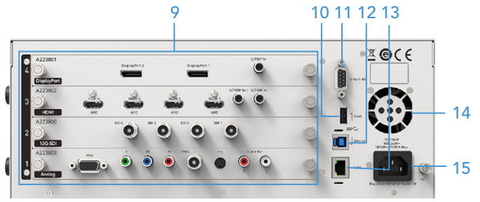
后背板
