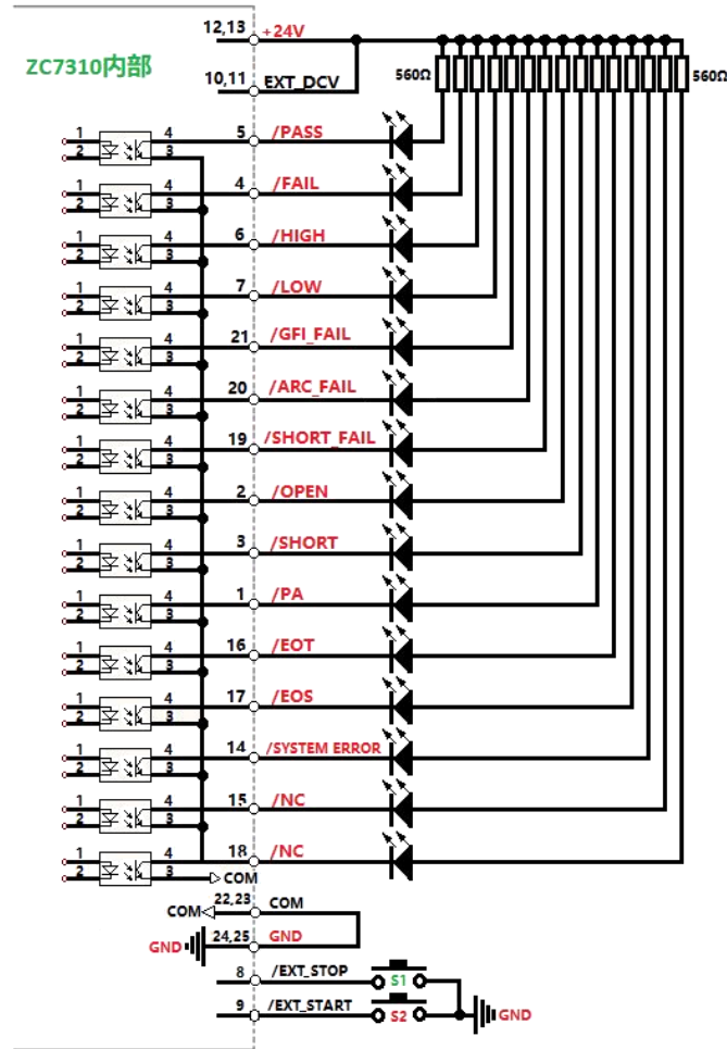
图 5.1.1.1 HANDLER 接口内部电源示意图
