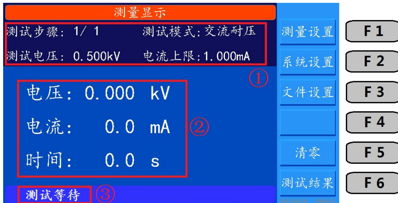
图 4.2.1 交流耐压测量显示界面
