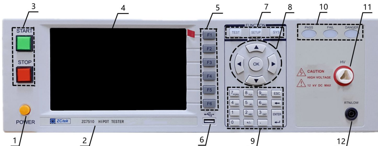
图 3-1 ZC7510 前面板示意图
