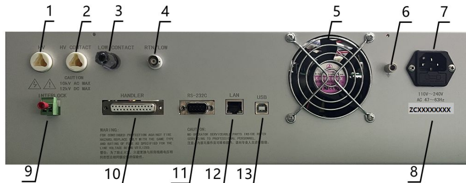
图 3-2 ZC7510 后面板示意图
