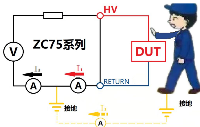
图 4.4.1 触电保护示意图
